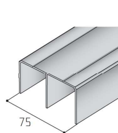
Profil S05
